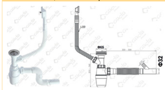
100114 - СИФОН БУТ.ПЛ./GP-ES0204У/С ВИТЛО- Ф65,ГОФРЕ-Ф32 и преливник
