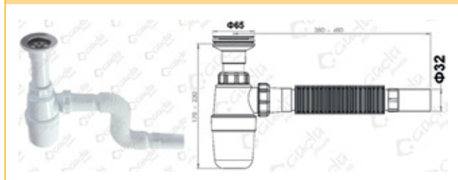
100111 - СИФОН БУТ.ПЛ./GP-LS0131/ С ВИТЛО-Ф65 И ГОФРЕ-Ф32
