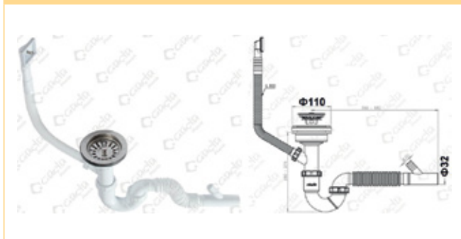
100114 - СИФОН БУТ.ПЛ./GP-ES0204Y/C ВИТЛО-Ф65,ГОФРЕ-Ф32 и преливник
